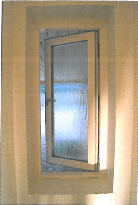
Udv BD30 vindue med råglas Brandtermoglas set inde og udefra
